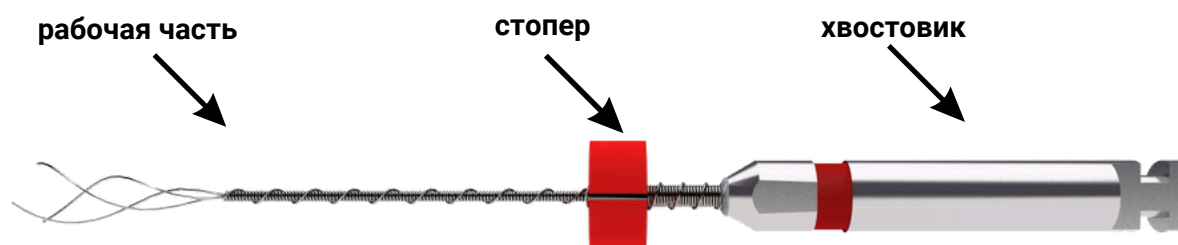
Рисунок 1 – Обозначение основных частей инструмент
